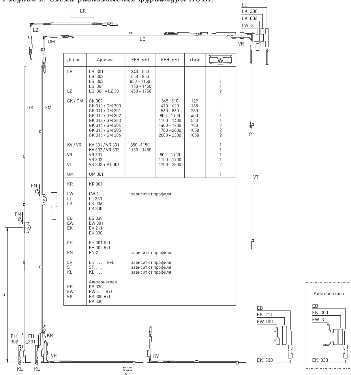
Рисунок 2. Схема расположения фурнитуры AUBI.
