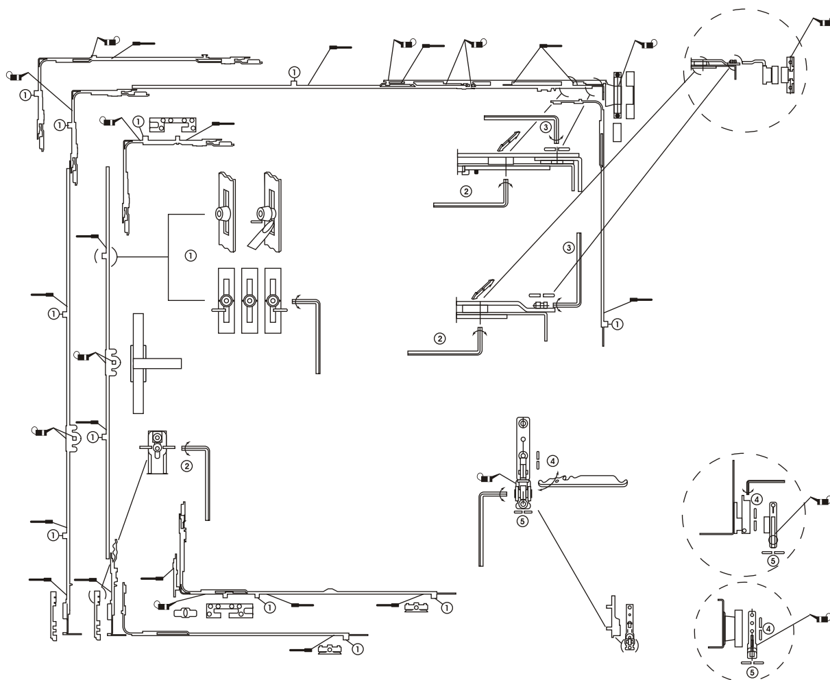
Рисунок 1. Схема регулировки и смазки фурнитуры AUBI.
