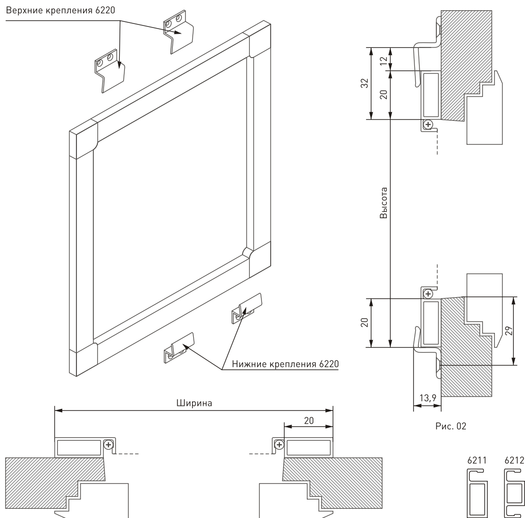
Рисунок 4. Противомоскитные сетки SKS – система PROFILIA для стандартных окон с выступающей рамой
