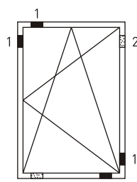
Поворотно-откидная створка
